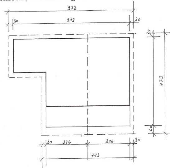
Dachform, Vermessung im Grund
