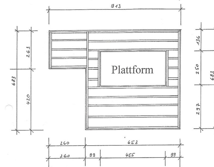
Balkenlage und Aussenmasse der Schwandistube
