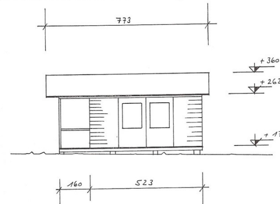
Längsansicht mit Höhenvermessung
